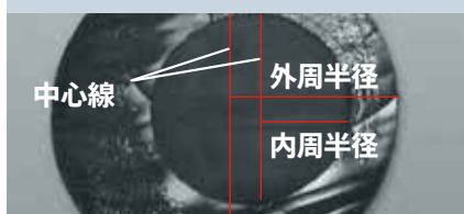
図3 不合格…中心線から のずれが許容公差 の0.75mm以内では ない
