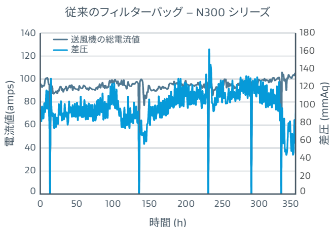
図1: 従来のフィルターバッグは、差圧が極めて高く、送風機の平均電流値と安定性はより低い傾向
