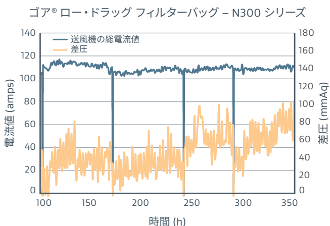
図2: ゴア ロー・ドラッグ フィルターバッグは差圧が一定して低い傾向を示すとともに、より高く一定した送風機電流値を実現
